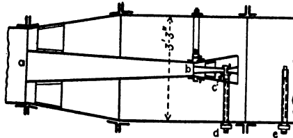
FIG. 103.—Rateau multiplier.
